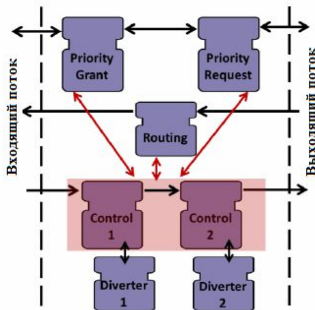
Рис. 5. Внутренняя структура соответствующего управляющего кода FB для конвейера с 2-мя фотоэлементами и 2-мя диверторами
