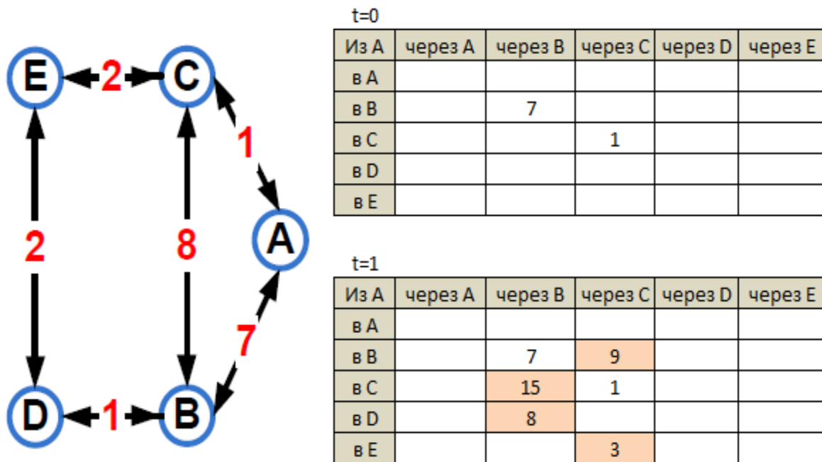
Рис. 6. Сеть из 5 маршрутизаторов с метриками расстояний и таблицами маршрутизации для узла A в момент времени t = 0 и t = 1
