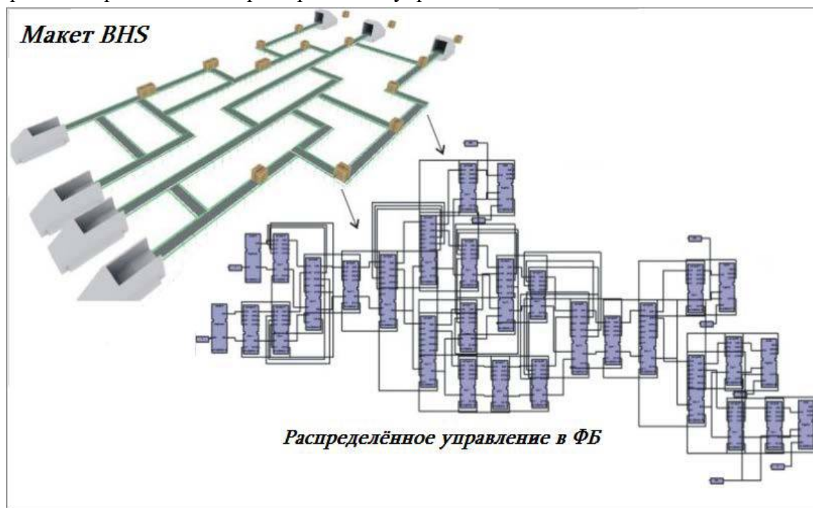
Рис. 3. Концепция дизайна BHS : от макета до децентрализованного управления и распределенного развертывания
