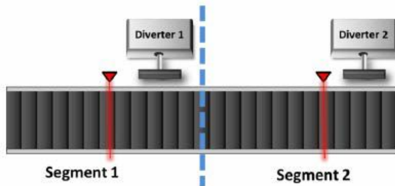
Рис. 4. Пример секции транспортера с двумя фоточувствительными датчиками и двумя диверторами
